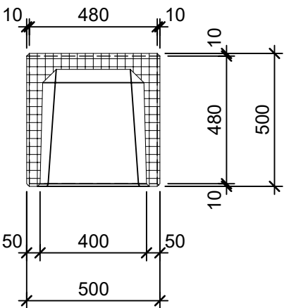
Schnitt 1-1 1:20
