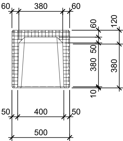
Schnitt 2-2 1:20
