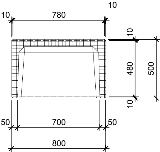
Schnitt 1-1 1:20
