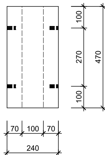
Grundriss 1:10
