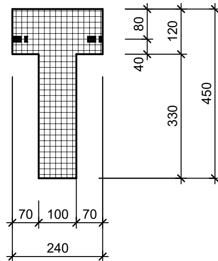
Schnitt 1:10
