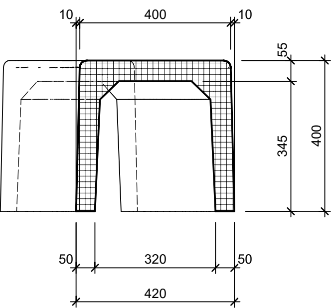
Schnitt 1-1 1:10
