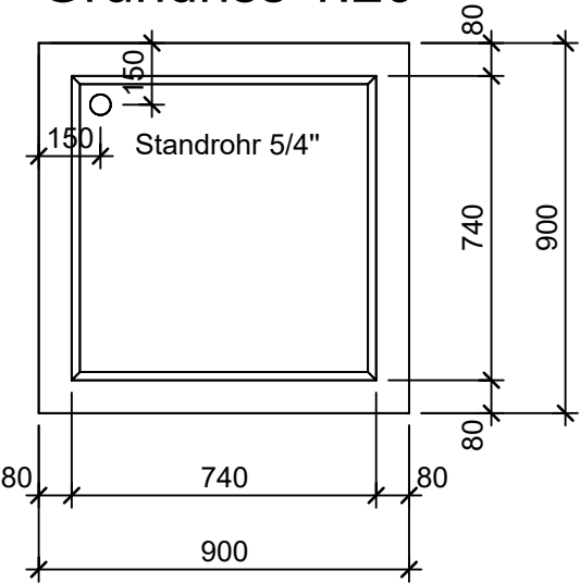
Grundriss 1:20
