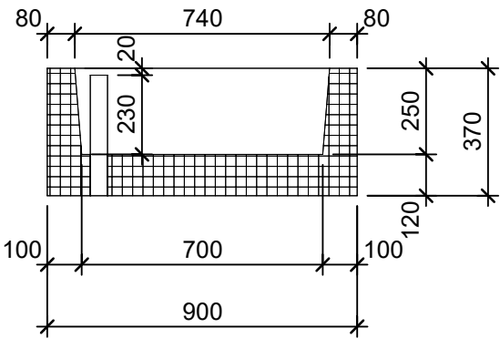
Schnitt 1-1 1:20
