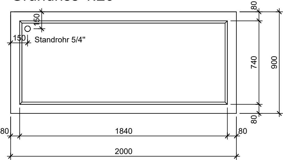
Grundriss 1:20
