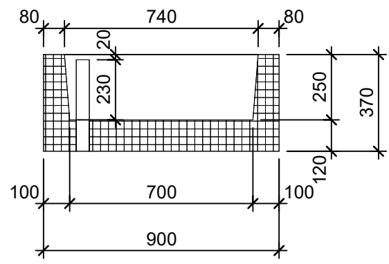
Schnitt 1-1 1:20
