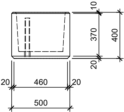
Ansicht 1:20
