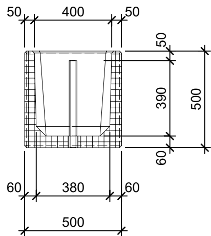
Schnitt 2-2 1:20
