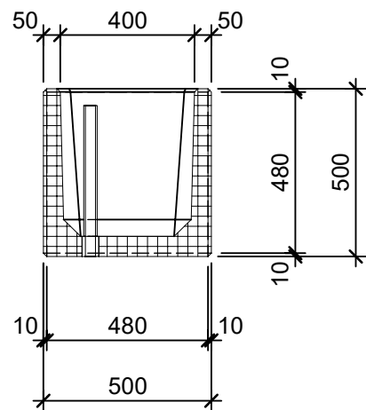
Schnitt 1-1 1:20
