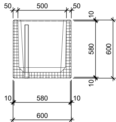
Schnitt 1-1 1:20
