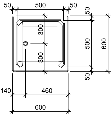
Grundriss 1:20
