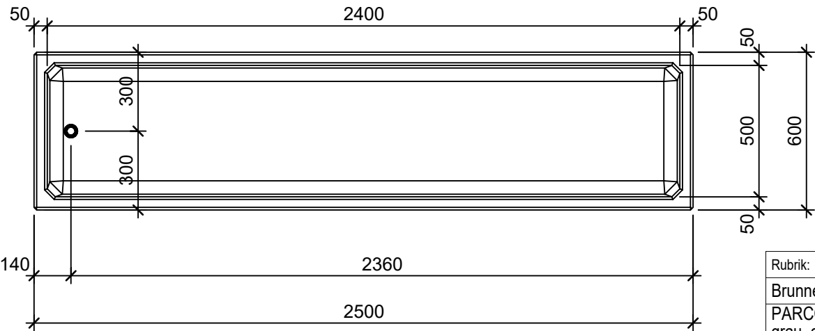
Grundriss 1:20
