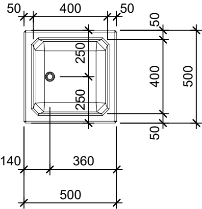
Grundriss 1:20
