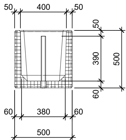
Schnitt 2-2 1:20
