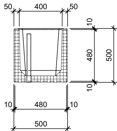
Schnitt 1-1 1:20
