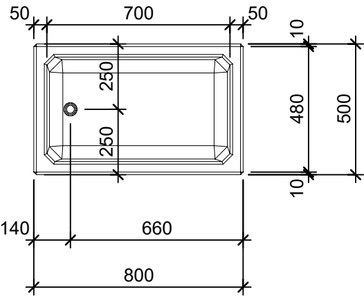
Grundriss 1:20
