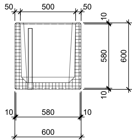
Schnitt 1-1 1:20
