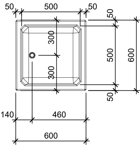
Grundriss 1:20
