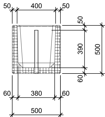
Schnitt 2-2 1:20
