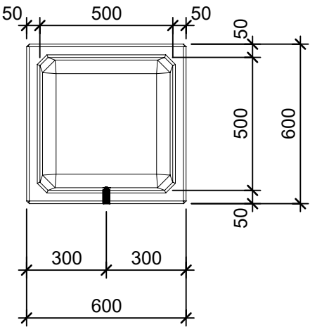
Grundriss 1:20
