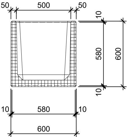
Schnitt 1-1 1:20
