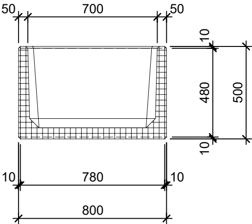
Schnitt 1-1 1:20
