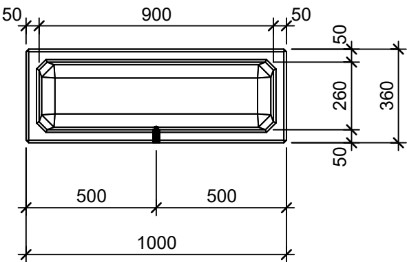
Grundriss 1:20
