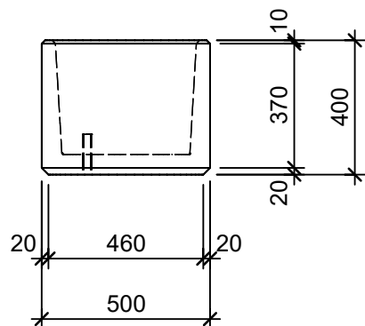
Ansicht 1:20
