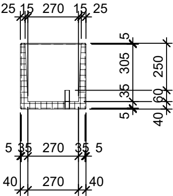
Schnitt 2-2 1:20
