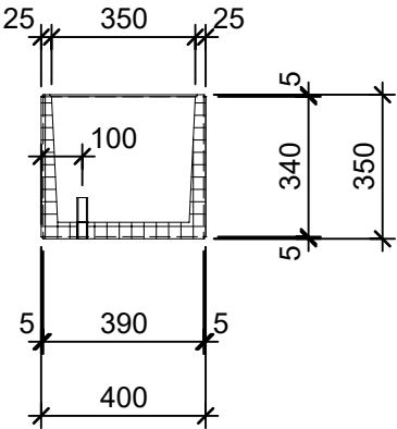
Schnitt 1-1 1:20
