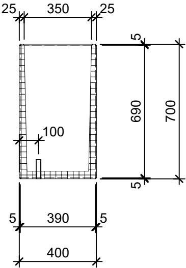
Schnitt 1-1 1:20
