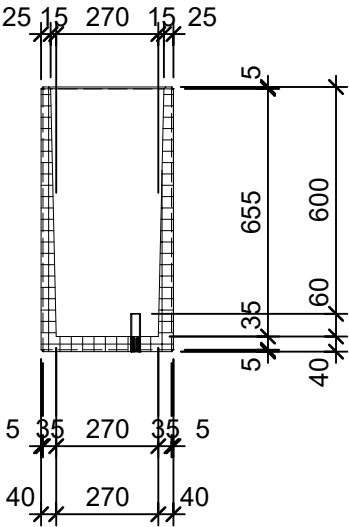
Schnitt 2-2 1:20
