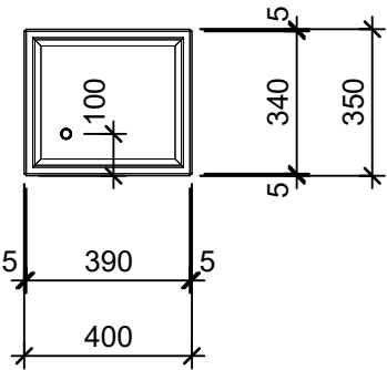
Grundriss 1:20
