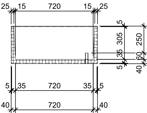
Schnitt 2-2 1:20
