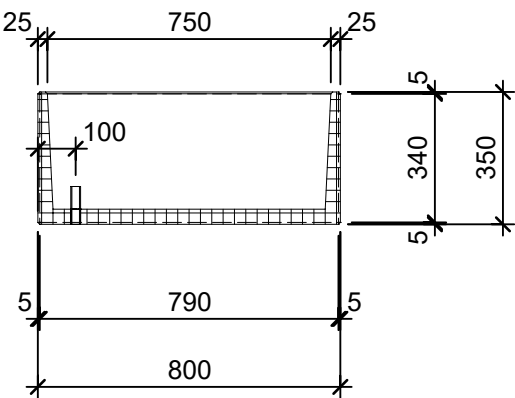
Schnitt 1-1 1:20
