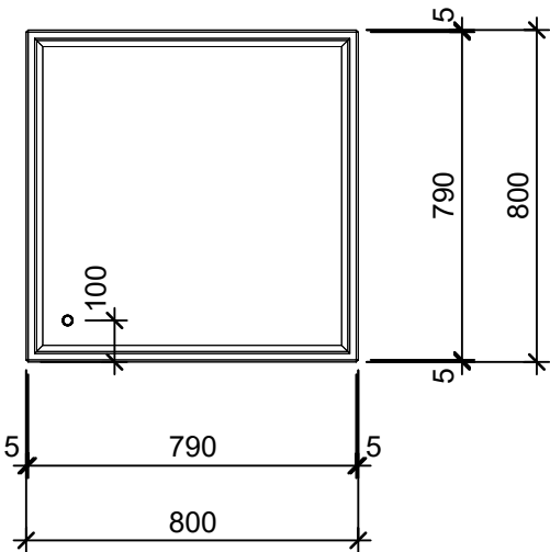
Grundriss 1:20
