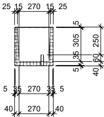
Schnitt 2-2 1:20
