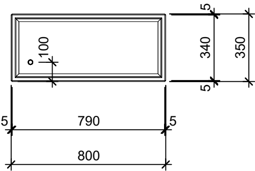
Grundriss 1:20
