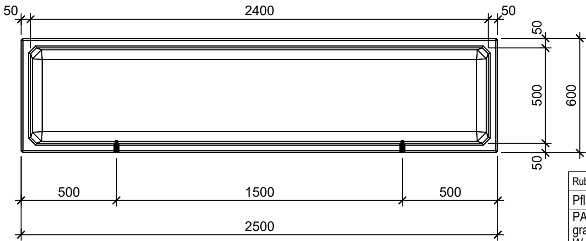
Grundriss 1:20
