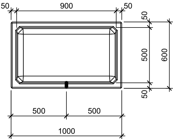
Grundriss 1:20
