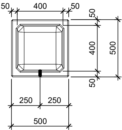
Grundriss 1:20
