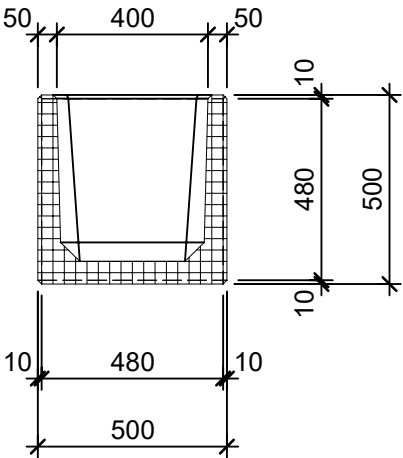
Schnitt 1-1 1:20
