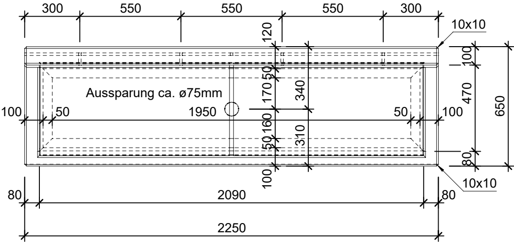
Grundriss 1:20
