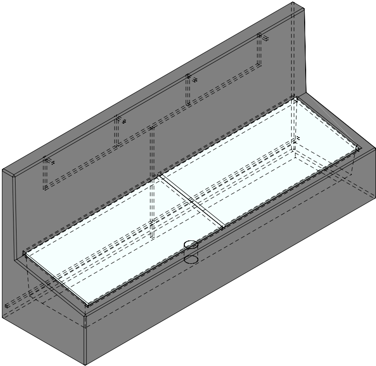
Isometrie 1:20
