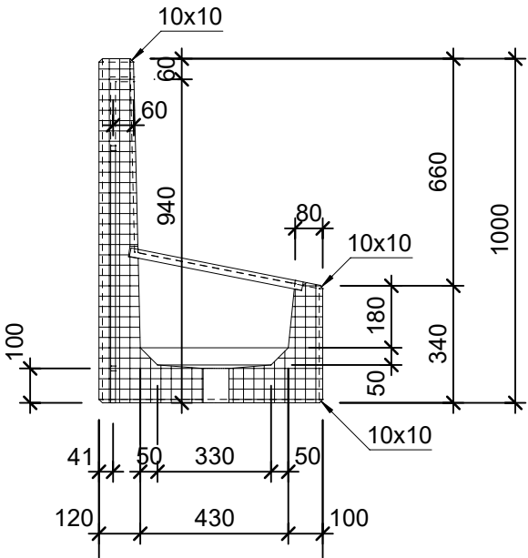
Schnitt 1-1 1:20
