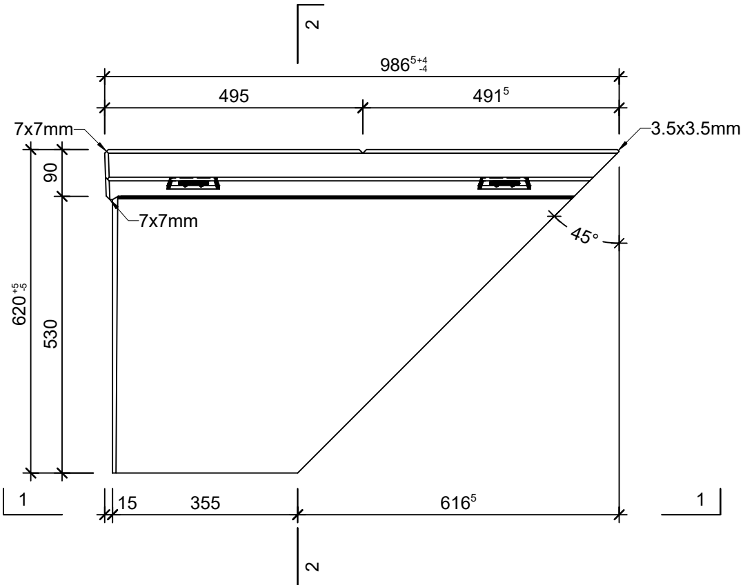
Grundriss, 1:10
