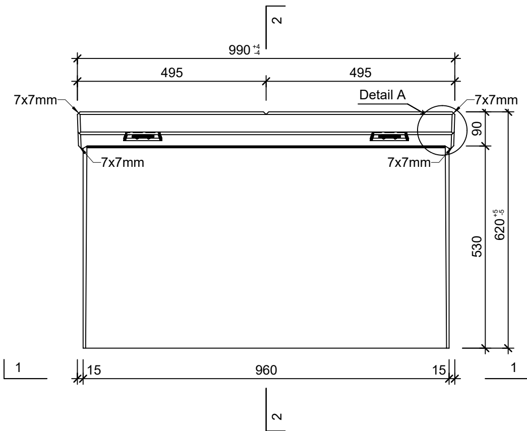
Grundriss, 1:10
