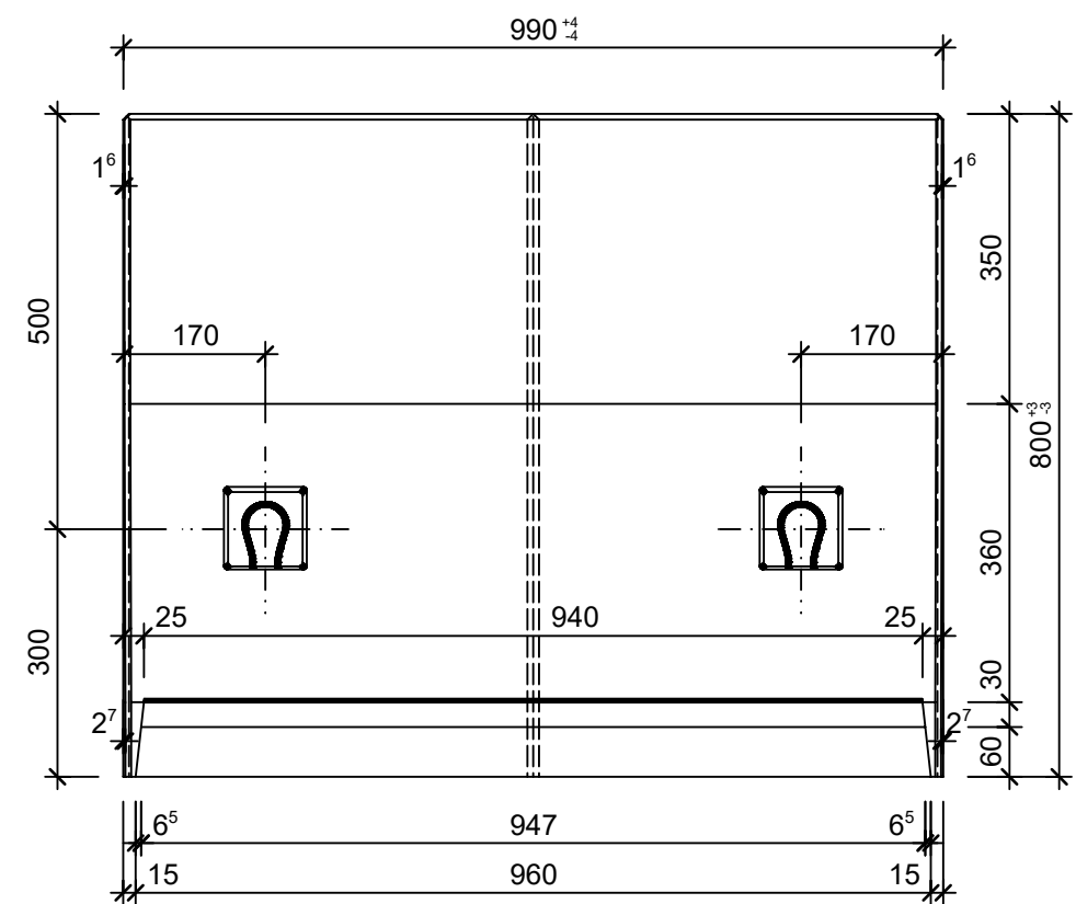
Grundriss, 1:10
