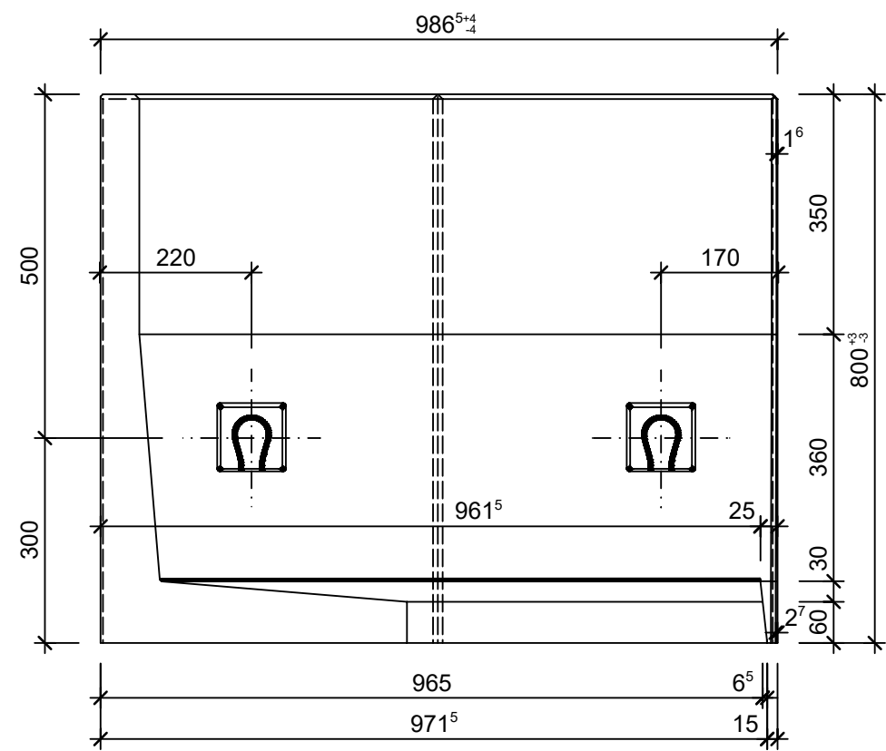
Grundriss, 1:10
