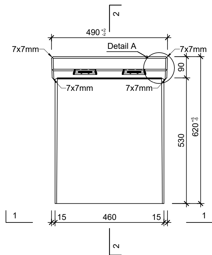
Grundriss, 1:10
