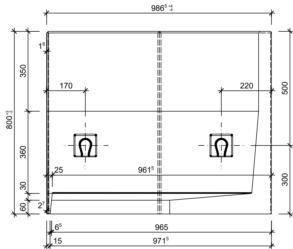
Grundriss, 1:10
