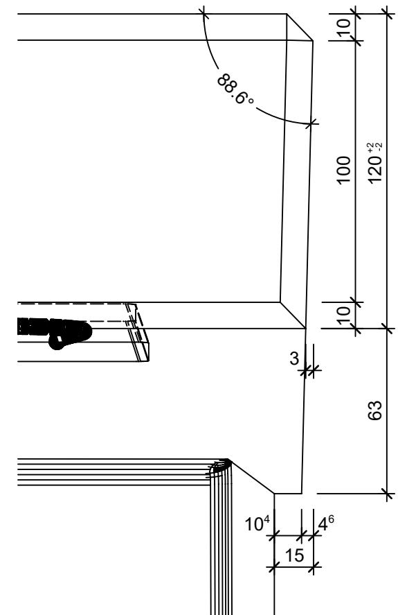
Detail A, 1:2
