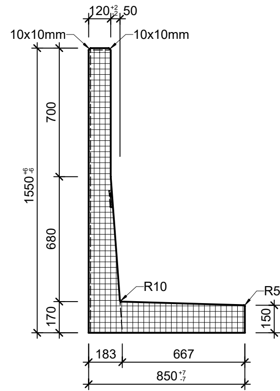
Schnitt 2-2, 1:20
