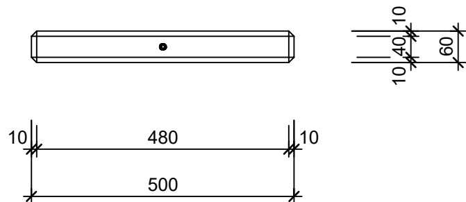
Grundriss 1:10
