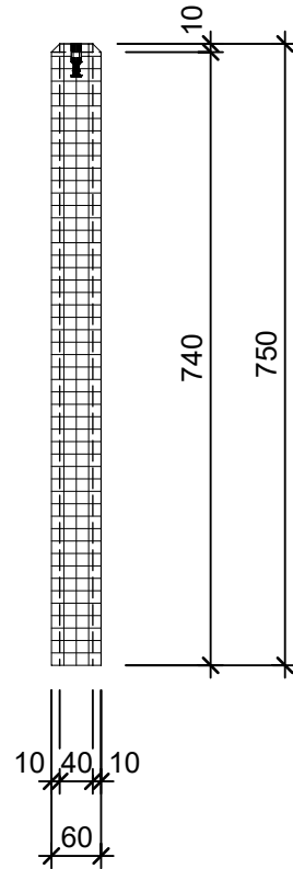
Schnitt 2-2 1:10
