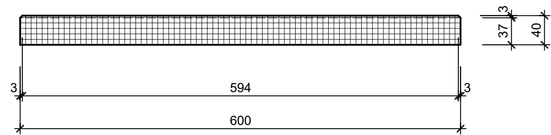
Schnitt 1-1 1:5
