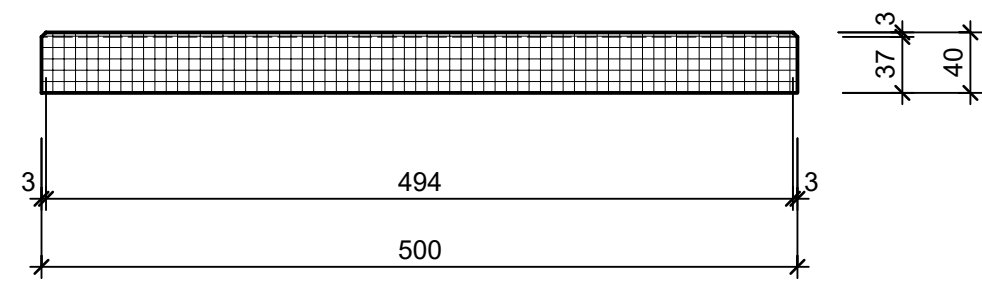
Schnitt 1-1 1:5
