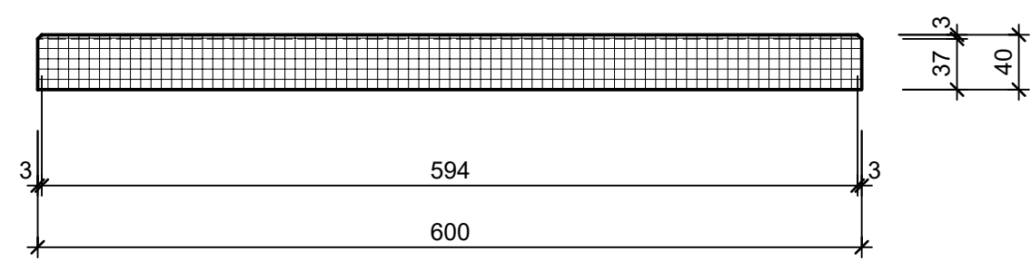
Schnitt 1-1 1:5
