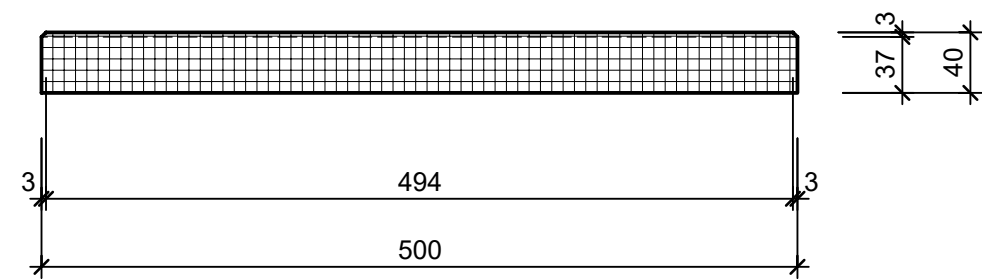
Schnitt 1-1 1:5
