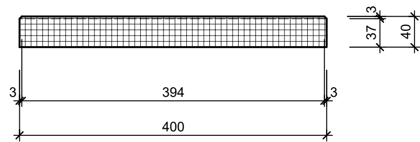
Schnitt 1-1 1:5
