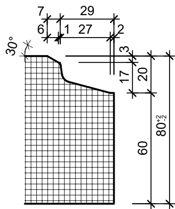
Schnitt 1-1, 1:2
