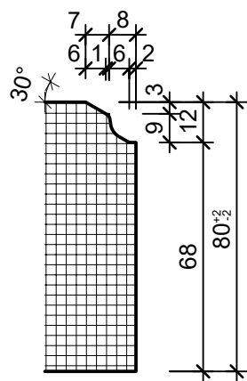
Schnitt 2-2, 1:2
