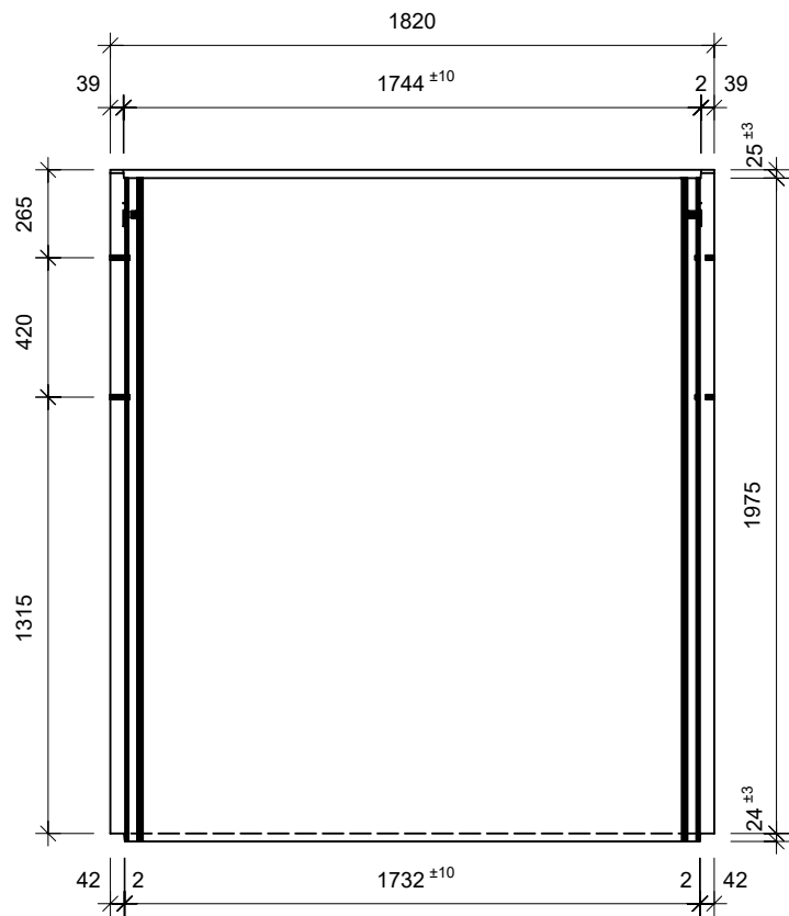
Ansicht 1-1, 1:25
