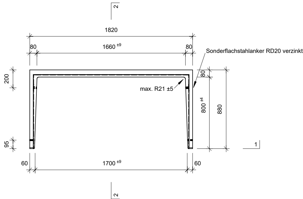
Grundriss, 1:25
