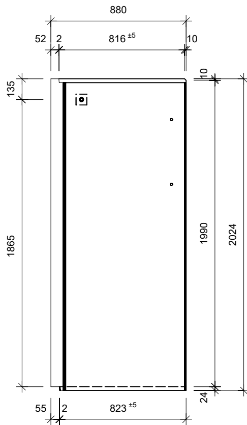
Schnitt 2-2, 1:25
