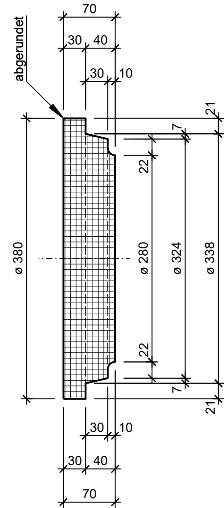
Schnitt B-B, 1:5
