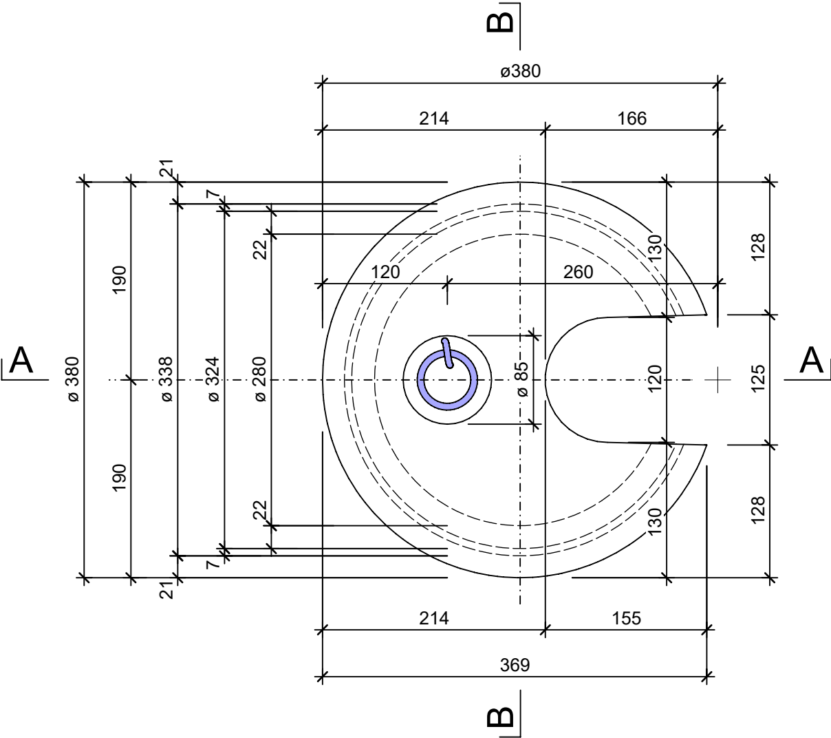
Grundriss, 1:5
