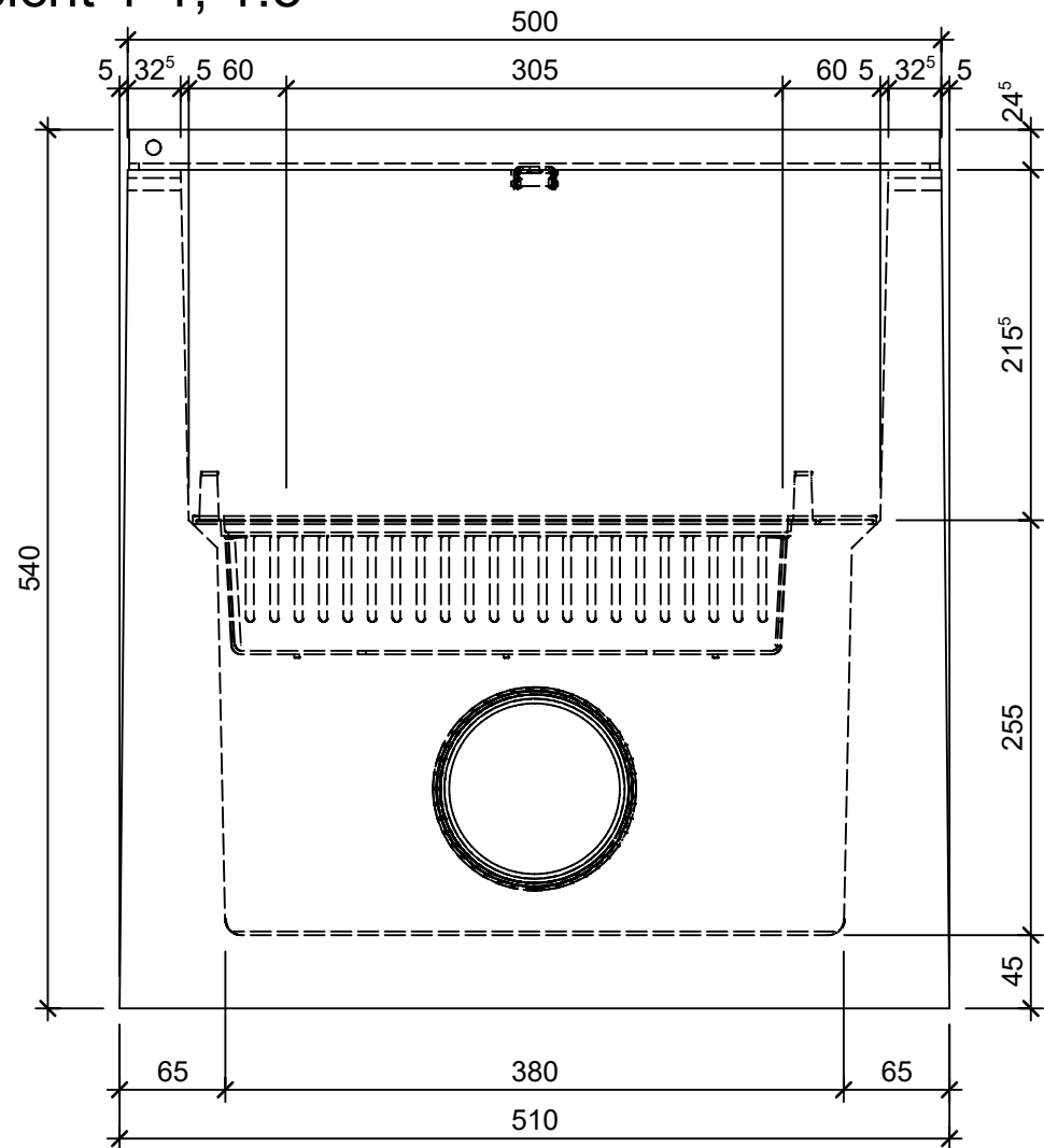
Ansicht 1-1, 1:5
