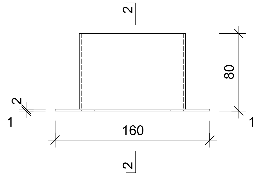
Grundriss, 1:2
