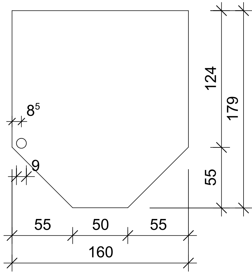
Ansicht 1-1, 1:2
