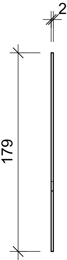
Schnitt 2-2, 1:2
