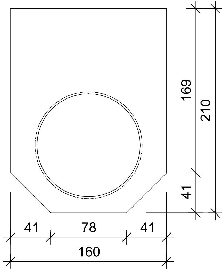
Ansicht 1-1, 1:2
