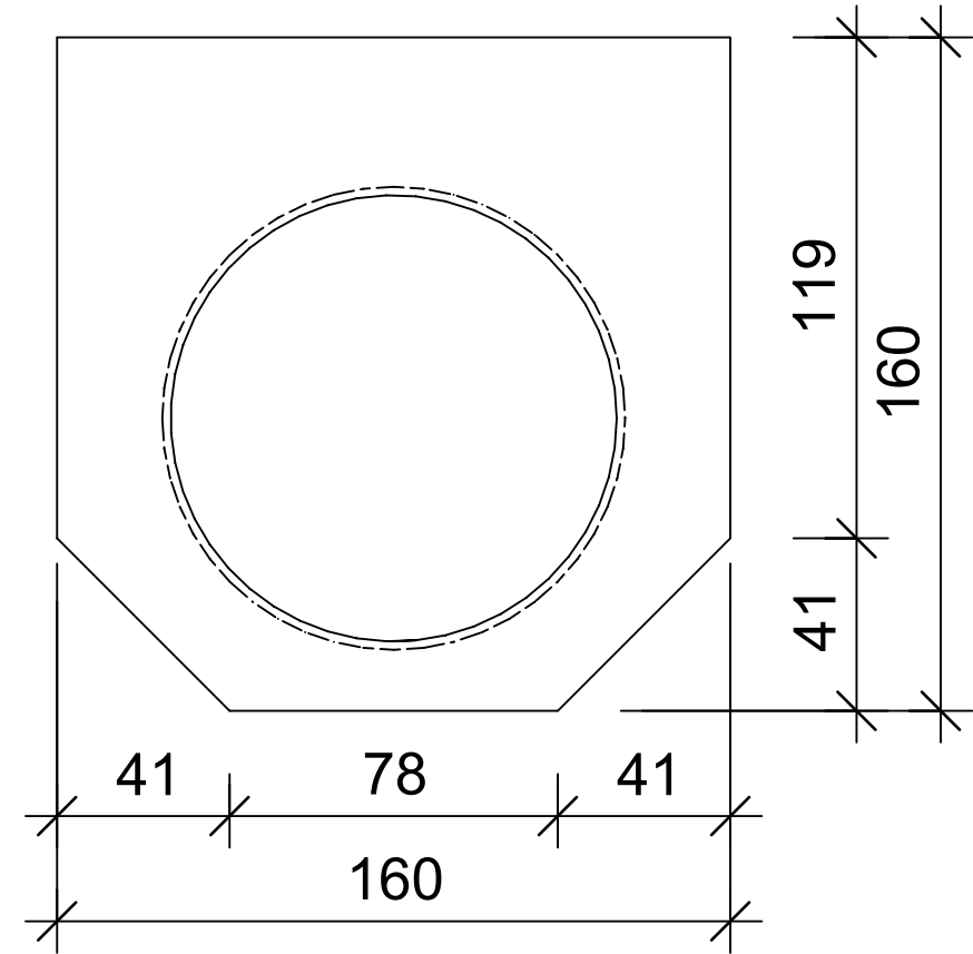
Ansicht 1-1, 1:2
