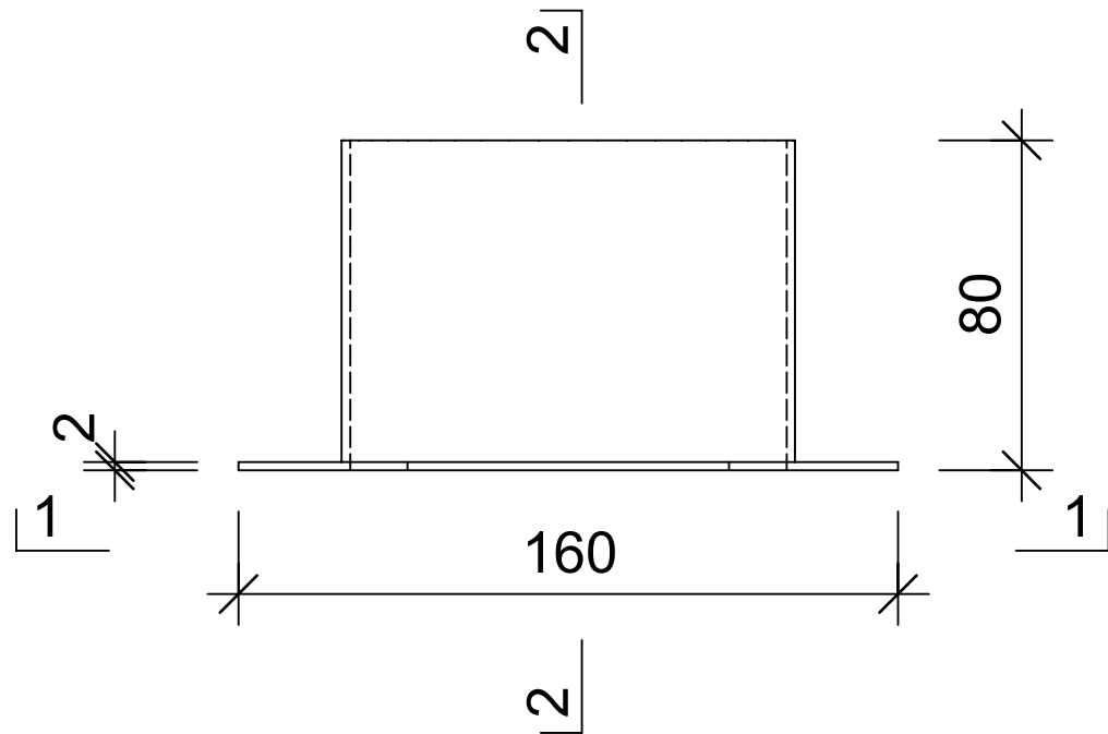
Grundriss, 1:2
