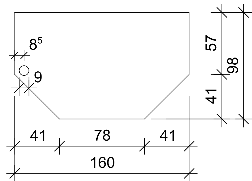
Grundriss, 1:2
