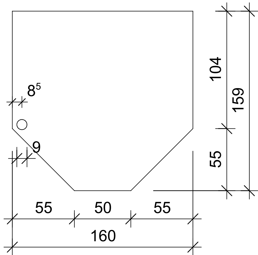
Ansicht 1-1, 1:2
