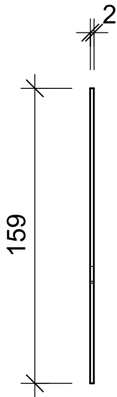
Schnitt 2-2, 1:2
