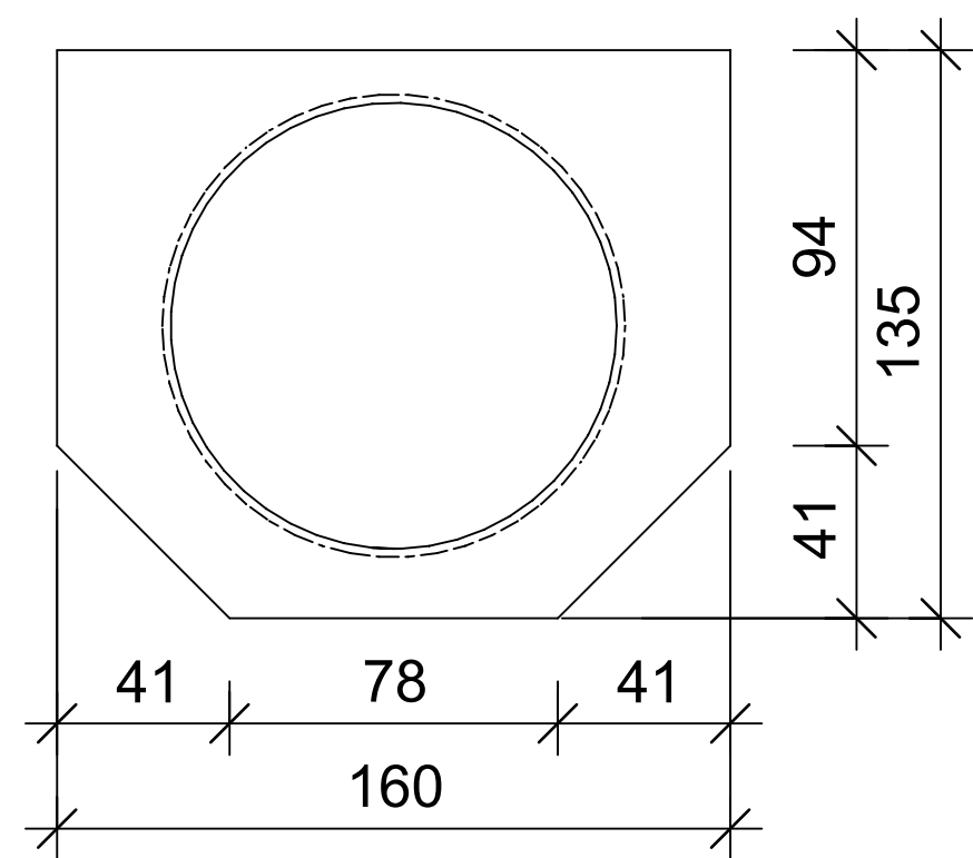
Grundriss, 1:2
