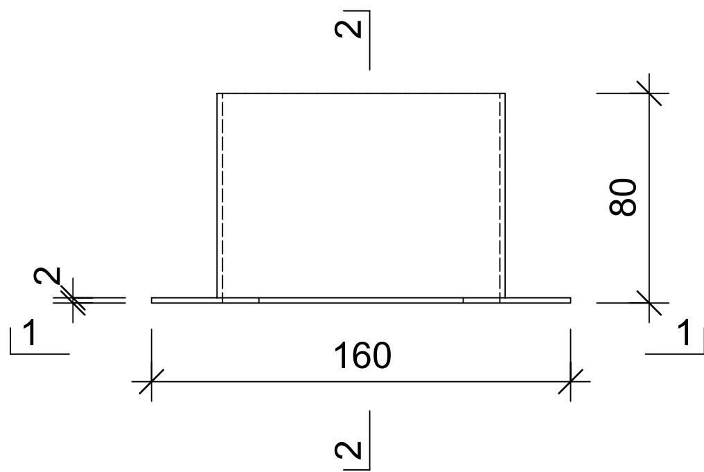
Grundriss, 1:2
